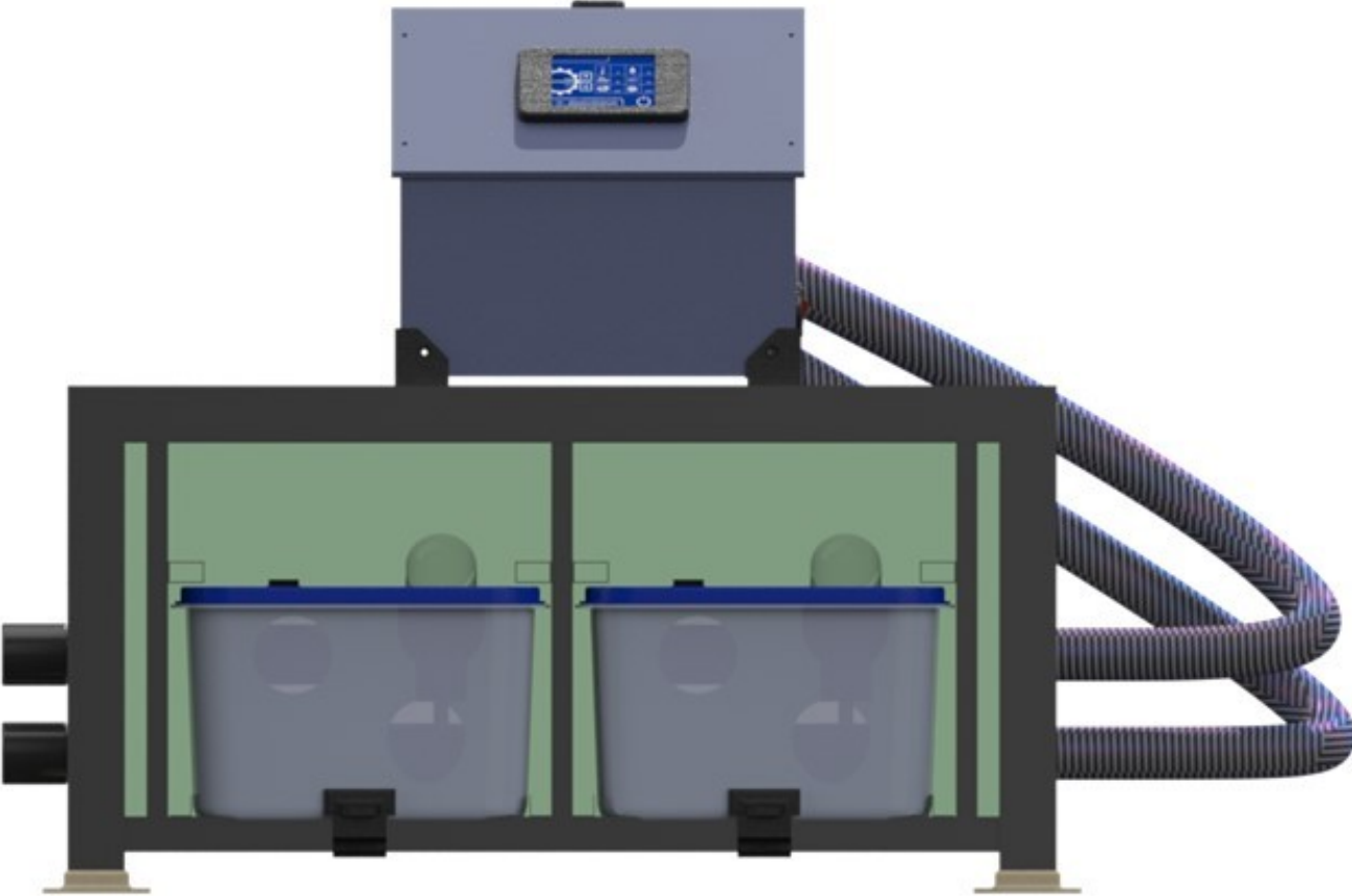
Gambar 2 - Tampak Depan
