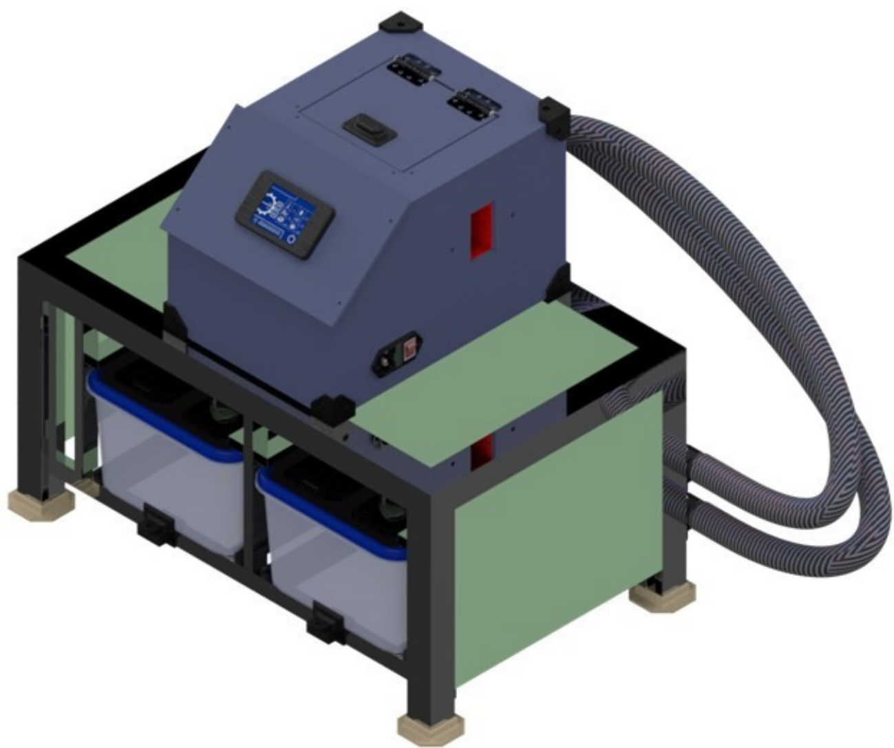
Gambar 1 - Tampak Perspektif
